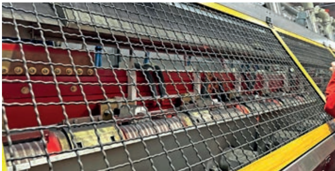
Die Stäbe werden erhitzt, wieder abgekühlt und erneut erhitzt. So erhalten sie genau definierte Festigkeits- und Zähigkeitseigenschaften.
